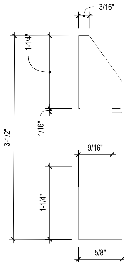
3 COUPE 1 Échelle: 1:1
