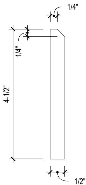
3 COUPE 1 Échelle: 1:2
