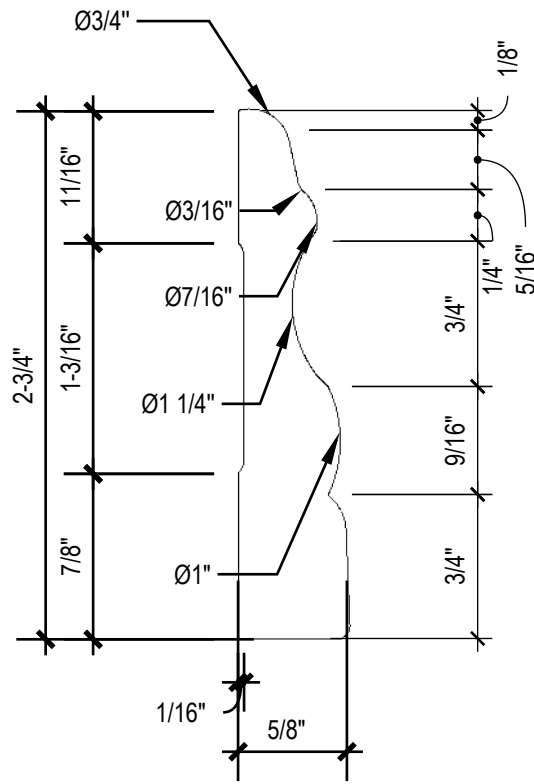
COUPE
