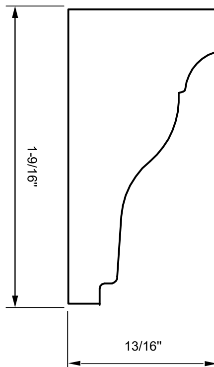
Vue de coupe modèle 113
