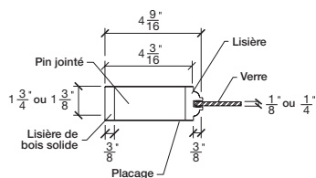
BATTANT
