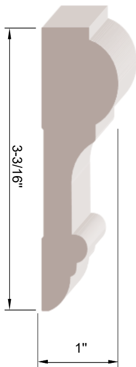
Vue de coupe modèle 103
